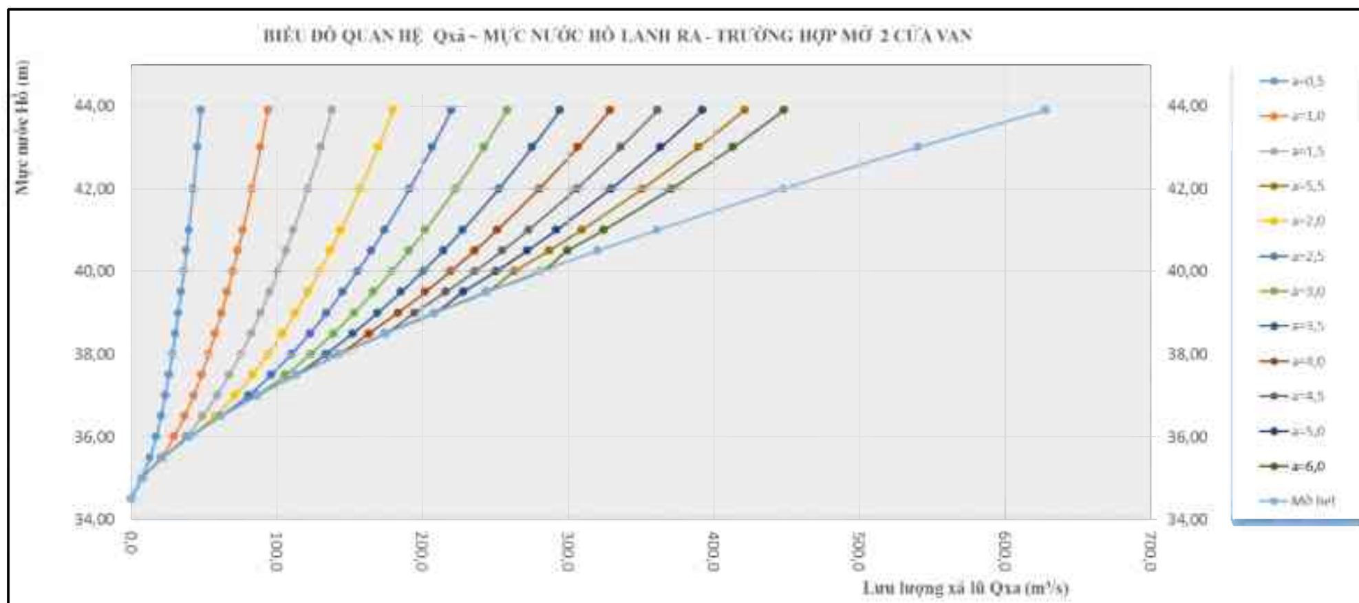
Hình PL 3.2: Lưu lượng qua tràn ~ Mức nước hồ ~ Độ mở cửa van (mở 2 cửa tràn)
