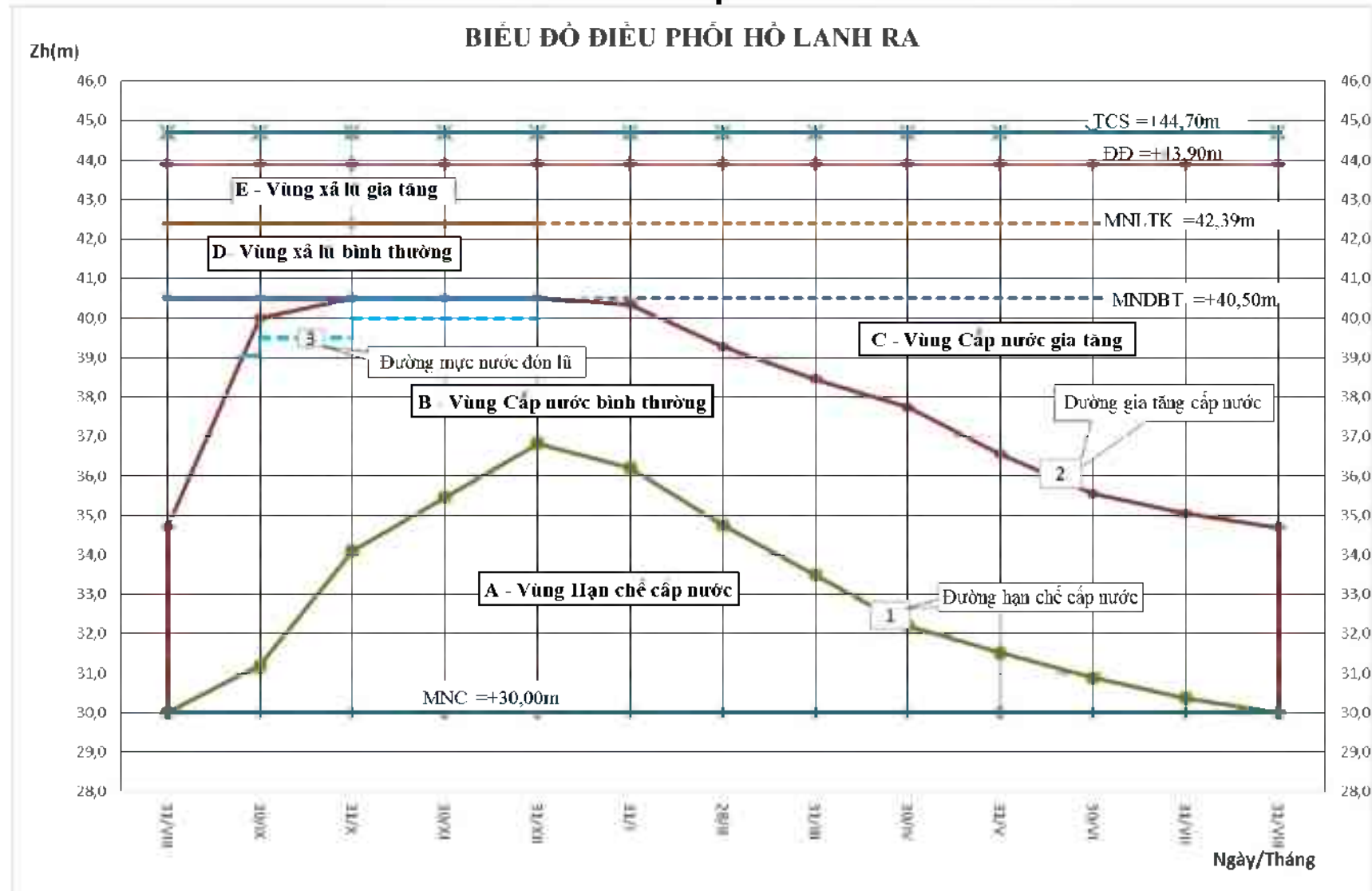
Hình PL5.1 Biểu đồ điều phối hồ chứa nước Lan Ra
