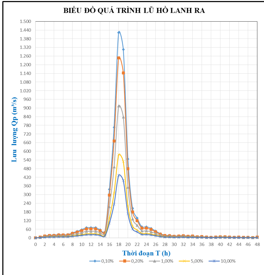
Hình PL 6.3 : Hình vẽ quá trình lũ đến hồ Lan Ra
