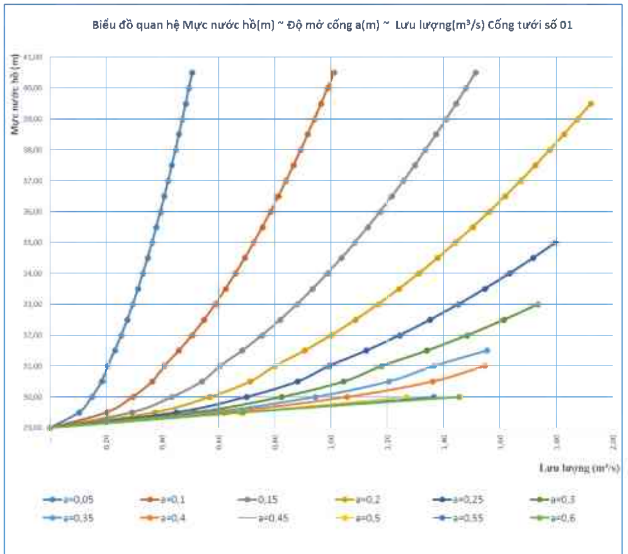
Hình PL4.1: Hình vẽ quan hệ mực nước hồ ~ Q xả công ~ Độ mở cổng lấy nước số 01 (m)
