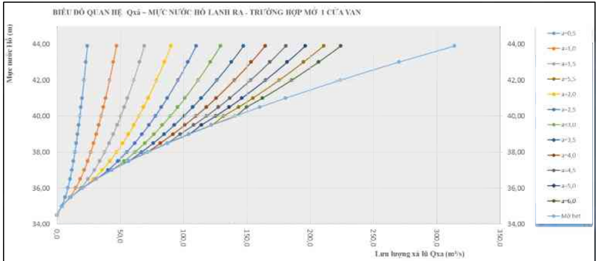
Hình PL 3.1: Lưu lượng qua tràn ~ Mức nước hồ ~ Độ mở cửa van (mở 1 cửa tràn)
