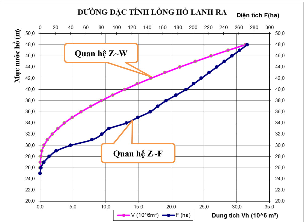
Hình PL2.1 Đường đặc tính hồ chứa nước Lanh Ra
